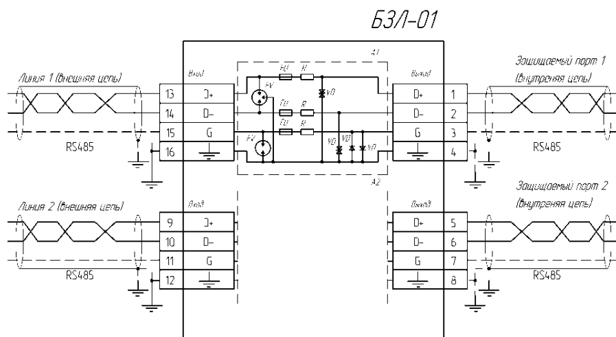
б) схема подключения
