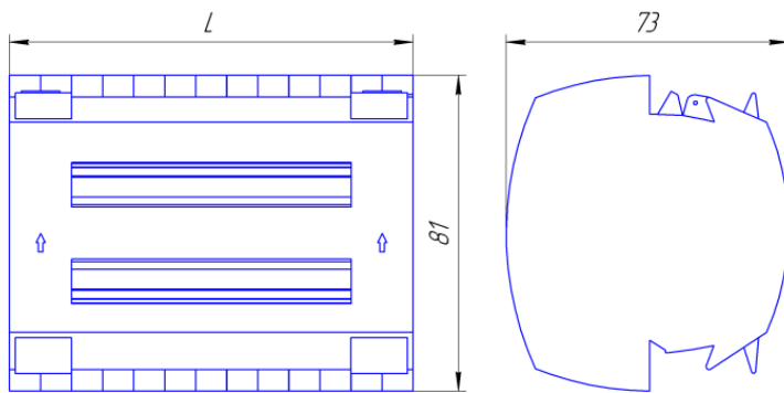
Рисунок 6 – Общий вид контрольной колодки с рабочей крышкой
