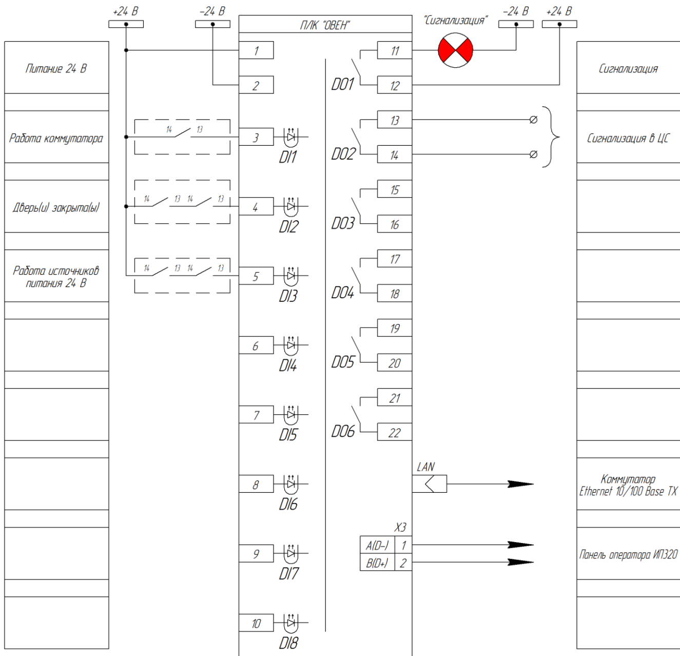
Рисунок 2 – Схема подключения ПЛК 100 «ОВЕН»
