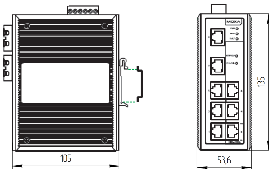
Рисунок 3 – Общий вид коммутаторов MOXA Ethernet Switch EDS-308 и EDS-408A
