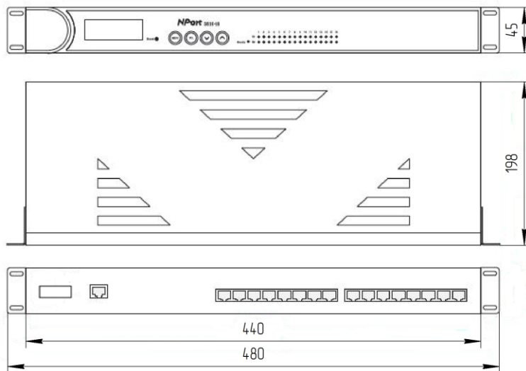
Рисунок 4 – Общий вид и назначение контактов последовательных портов сервера портов MOXA NPort 5650-16(8)
