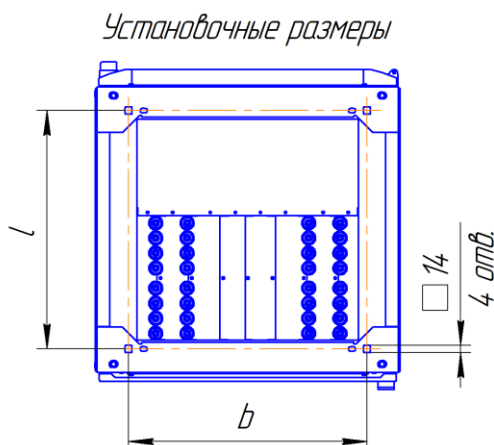
Рисунок 7 – Габаритные и установочные размеры шкафа
